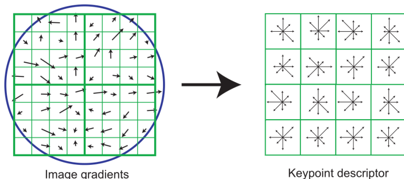
Image gradients
